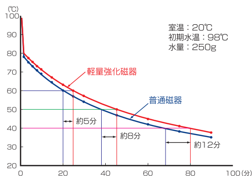
普通磁器と軽量強化磁器の保温性(当社比)
